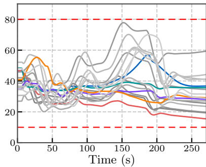
RNDDPC
